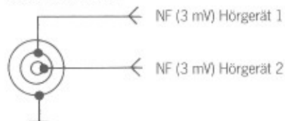
Abb. 3: Beschaltung der NF Ausgangsbuchse in Schalterstellung „3 mV“
